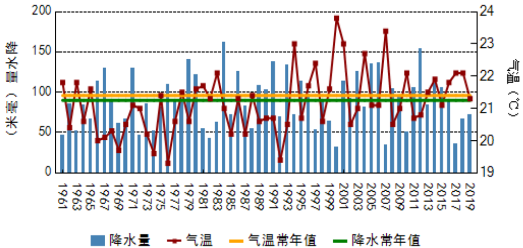
图1 辽宁省6月降水量、气温年际变化图
