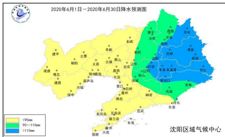
图2 2020年6月辽宁降水量预测图(单位: mm)
