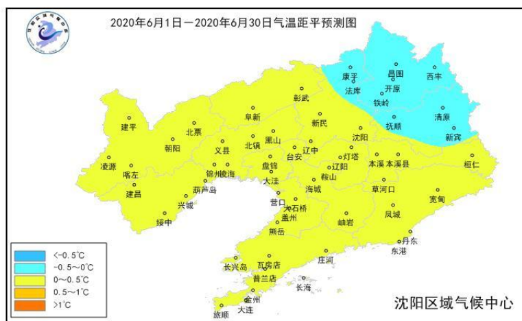
图4 2020年6月辽宁气温距平预测图（单位：℃）
