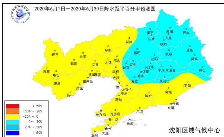
图3 2020年6月辽宁降水距平百分率预测图（单位：%）
